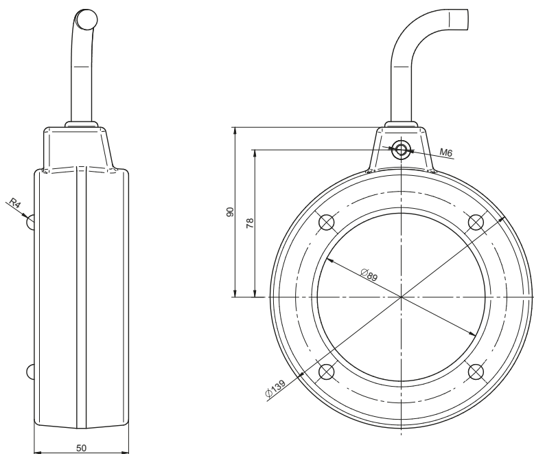
Wymiary gabarytowe
