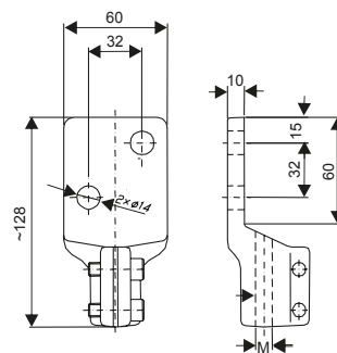
Odwiercenie zacisku zgodne z BN-76/3071-72
