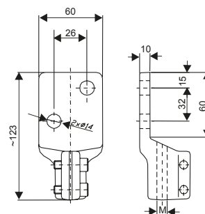
Odwiercenie zacisku zgodne z BN-76/3071-72
