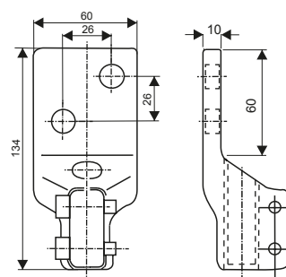
Odwiercenie zacisku zgodne z DIN4253269
