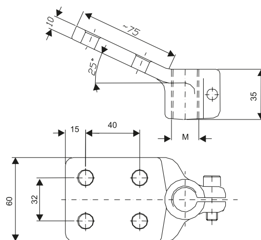
Możliwość połączenia szyn pod kątem 25°
