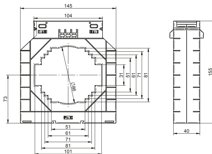
Wymiary gabarytowe
